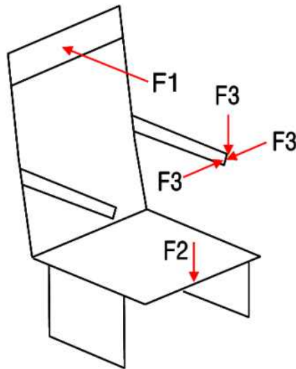
그림 1. 객실의자의 정하중 작용 기준
