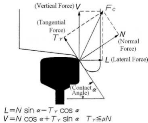
그림 1. Interaction forces between wheel and rail
