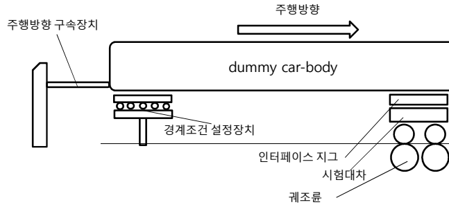
그림 2. 시험체 구성 개략도
