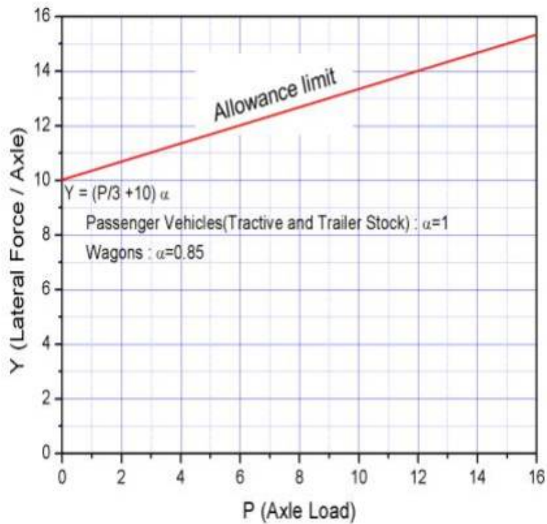
그림 4. 횡압 허용한도
