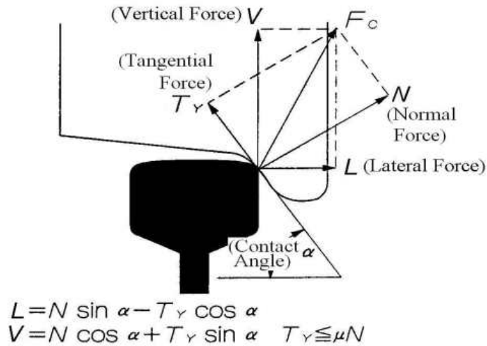
그림 1. Interaction forces between wheel and rail
