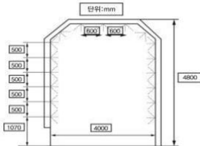
그림 1. 살수장치의 예시
