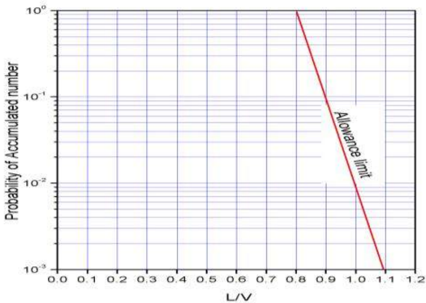
그림 3. 탈선계수 허용한도
