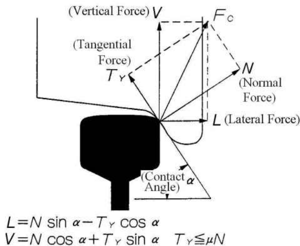
그림 1. Interaction forces between wheel and rail
