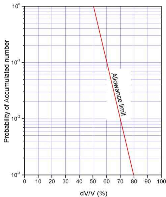
그림 5. 윤중감소율 허용한도
