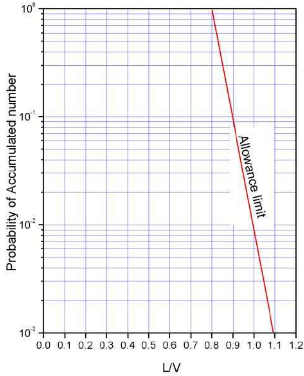
그림 3. 탈선계수 허용한도
