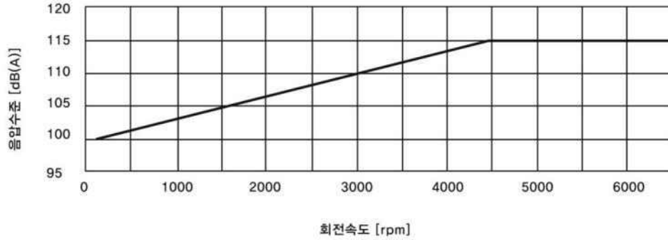
그림 4. 소음한계 기준치
