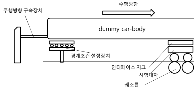
그림 2. 시험체 구성 개략도
