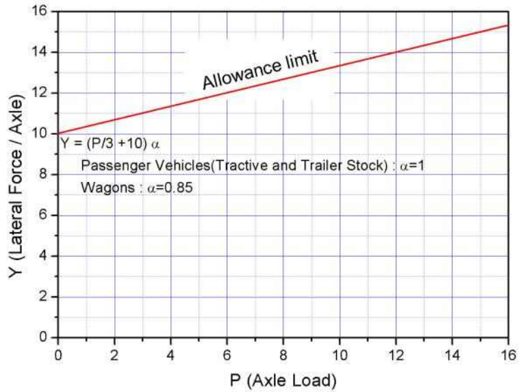
그림 4. 횡압 허용한도
