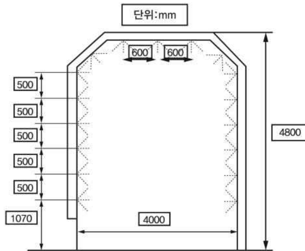
그림 1. 살수장치의 예시
