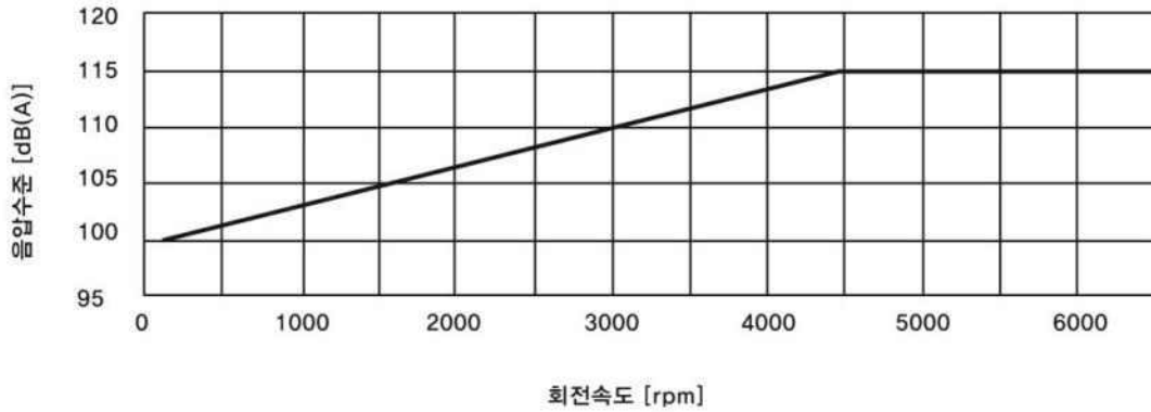
그림 4. 소음한계 기준치
