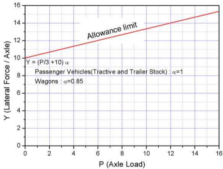
그림 4. 횡압 허용한도
