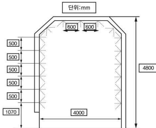
그림 1. 살수장치의 예시
