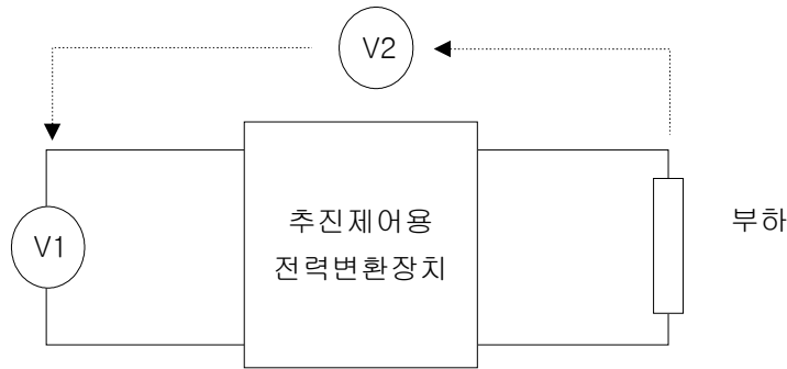
그림 2. 온도상승시험 회로구성
