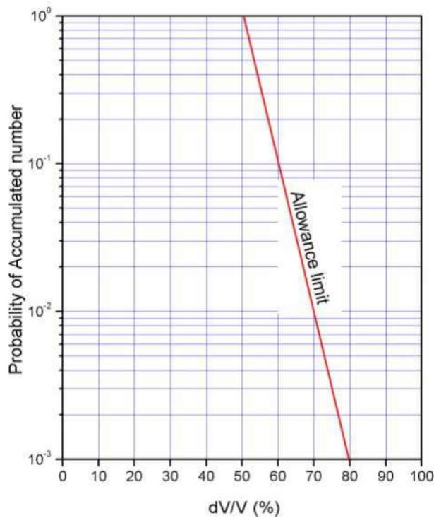
그림 5. 윤중감소율 허용한도
