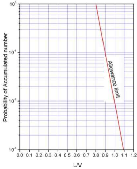
그림 3. 탈선계수 허용한도
