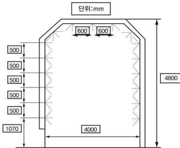
그림 1. 살수장치의 예시
