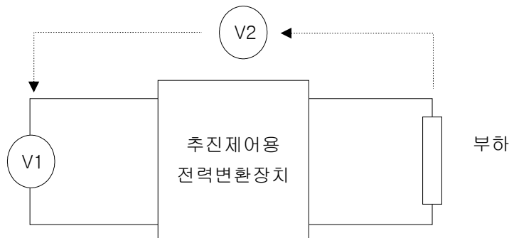
그림 1. 온도상승시험 회로구성
