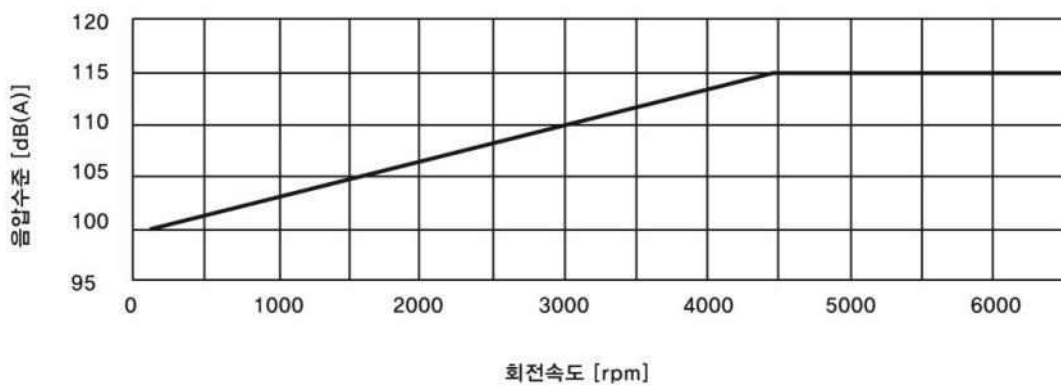
그림 3. 소음한계 기준치
