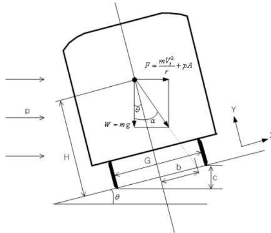
<그림 1> 차량의 중심선과 합력의 작용점
