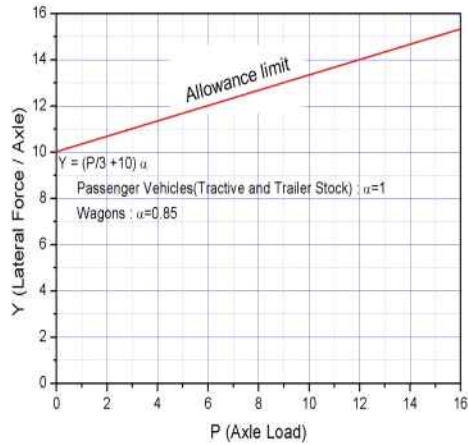
그림 4. 횡압 허용한도
