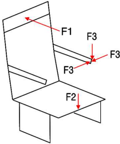
그림 1. 객실의자의 정하중 작용 기준
