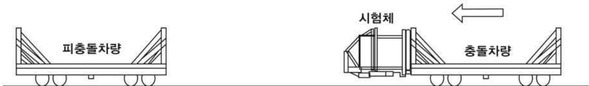
그림 2 차대차 충돌시험 개략도
