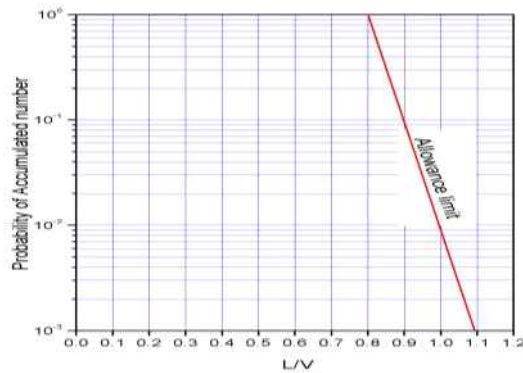
그림 3. 탈선계수 허용한도
