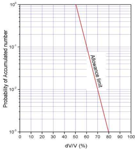
그림 5. 윤중감소율 허용한도
