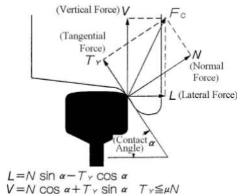
그림 1. Interaction forces between wheel and rail
