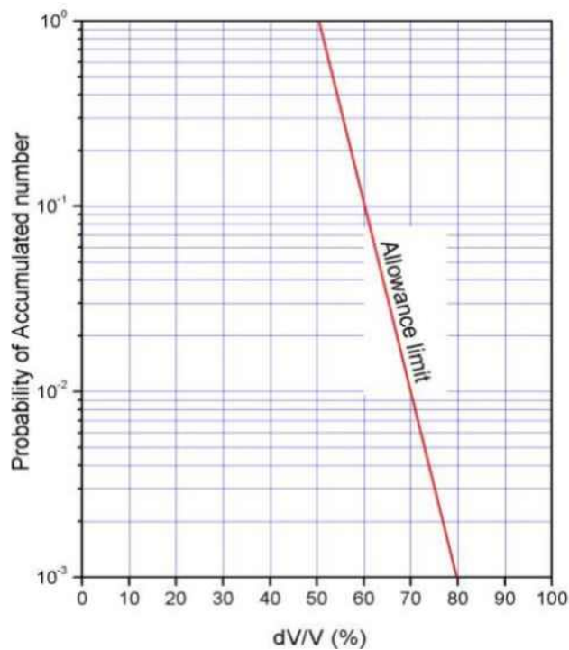
그림 5. 윤중감소율 허용한도
