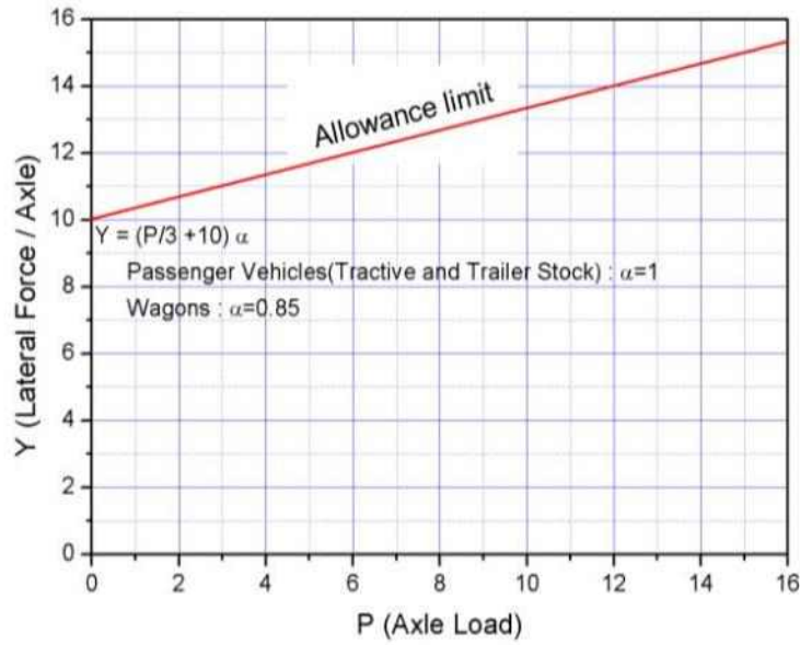
그림 4. 횡압 허용한도
