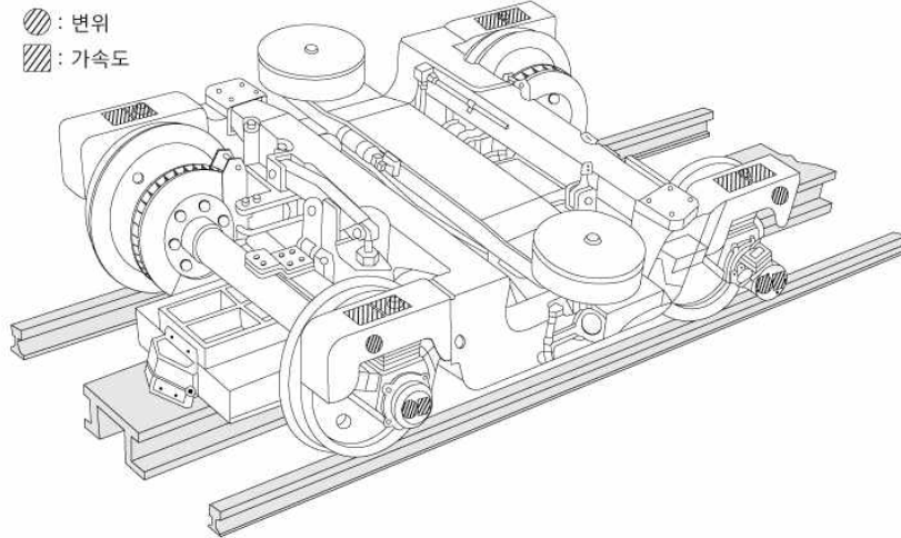
그림 3. 측정위치
