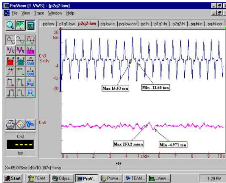
그림 2. Example of pulse (V, L)
