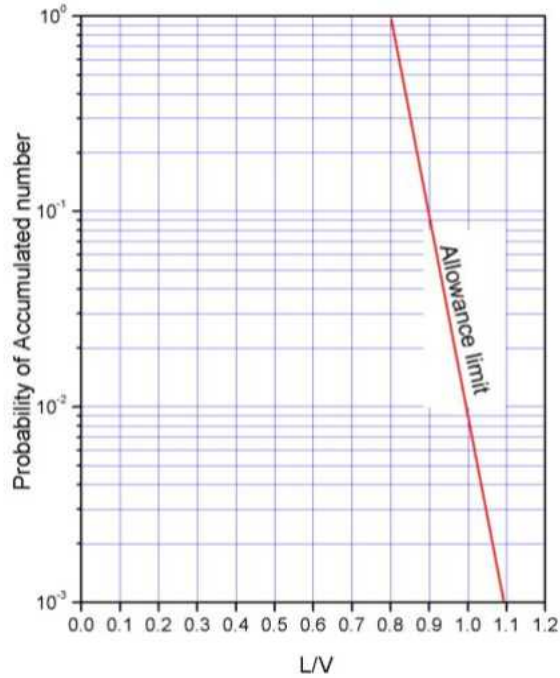
그림 3. 탈선계수 허용한도
