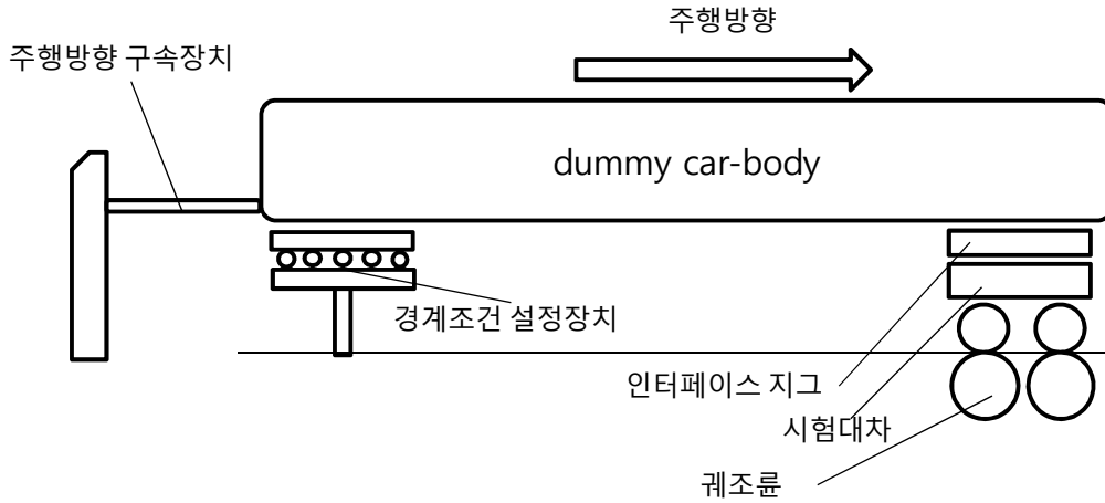
그림 2. 시험체 구성 개략도
