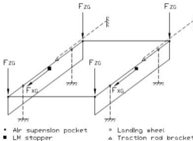
그림 6. 착지주행 전후하중시험의 대차 고정 및 하중 부가
