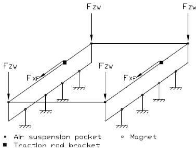
그림 12. 전자석 흡착 하중시험의 대차 고정 및 하중 부가
