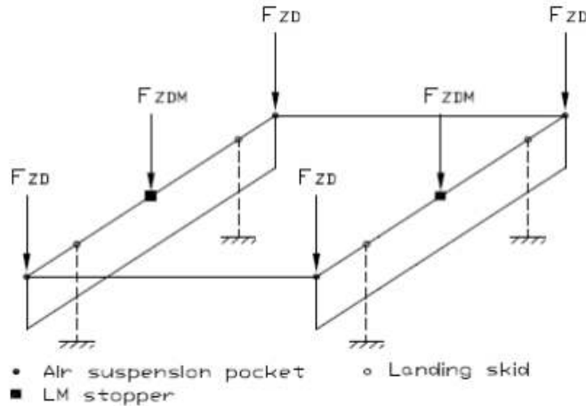
그림 13. 비틀림 하중시험의 대차 고정 및 하중 부가
