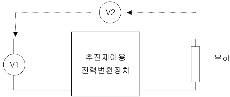
그림 1. 온도상승시험 회로구성
