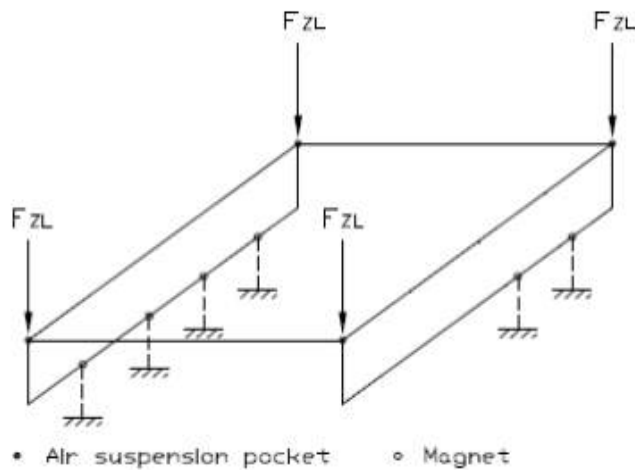
그림 10. 비틀림 하중시험의 대차 고정 및 하중 부가
