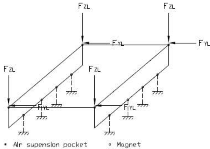
그림 3. 부상주행 좌우하중시험의 대차 고정 및 하중 부가
