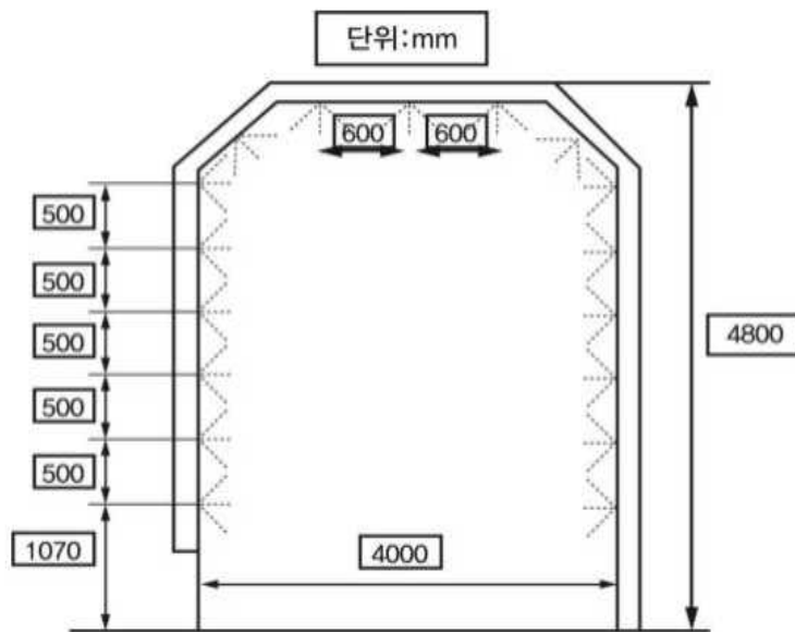
그림 1. 살수장치의 예시
