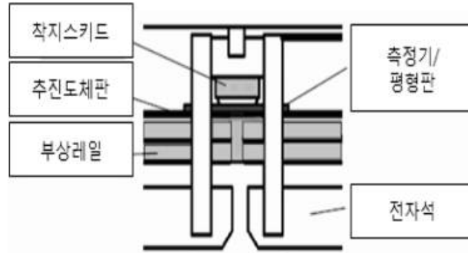
그림 1. 레일 상면에서의 차량 중량측정 예
