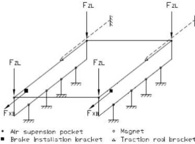
그림 11. 제동 하중시험의 대차 고정 및 하중 부가
