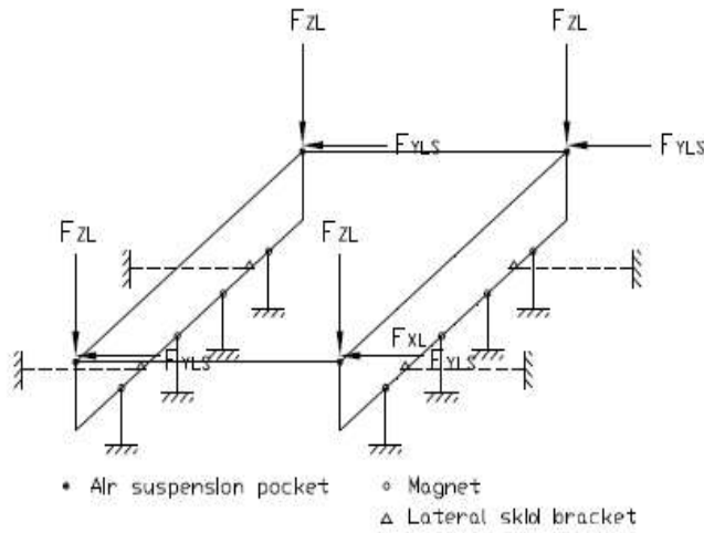
그림 7. 부상주행 안내스키드 하중시험의 대차 고정 및 하중 부가
