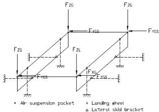
그림 8. 착지주행 안내스키드 하중시험의 대차 고정 및 하중 부가
