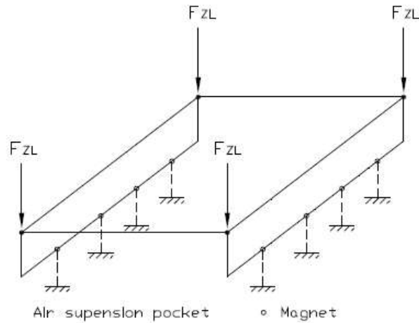
그림 1. 부상주행 수직하중시험의 대차 고정 및 하중 부가
