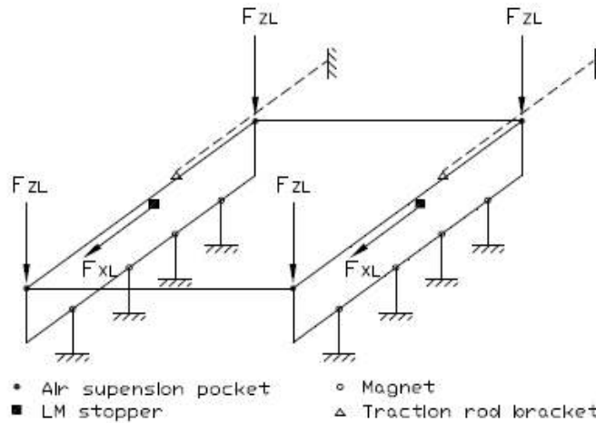
그림 5. 부상주행 전후하중시험의 대차 고정 및 하중 부가
