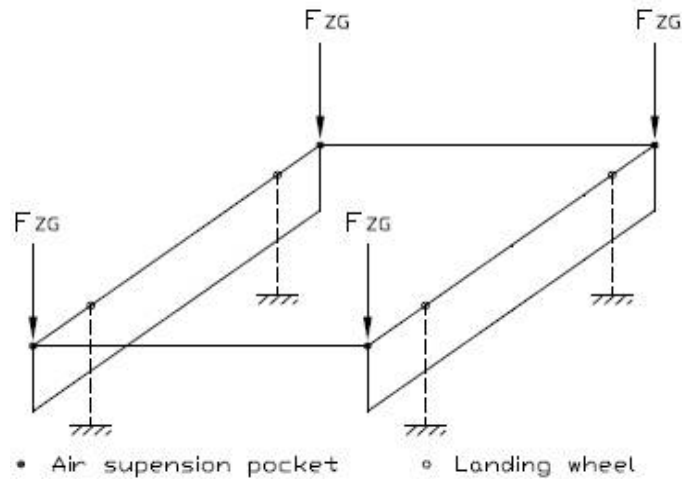
그림 2. 착지주행 수직하중시험의 대차 고정 및 하중 부가
