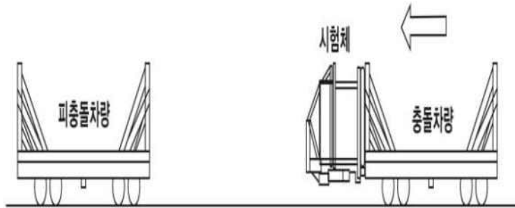
그림 2 차대차 충돌시험 개략도
