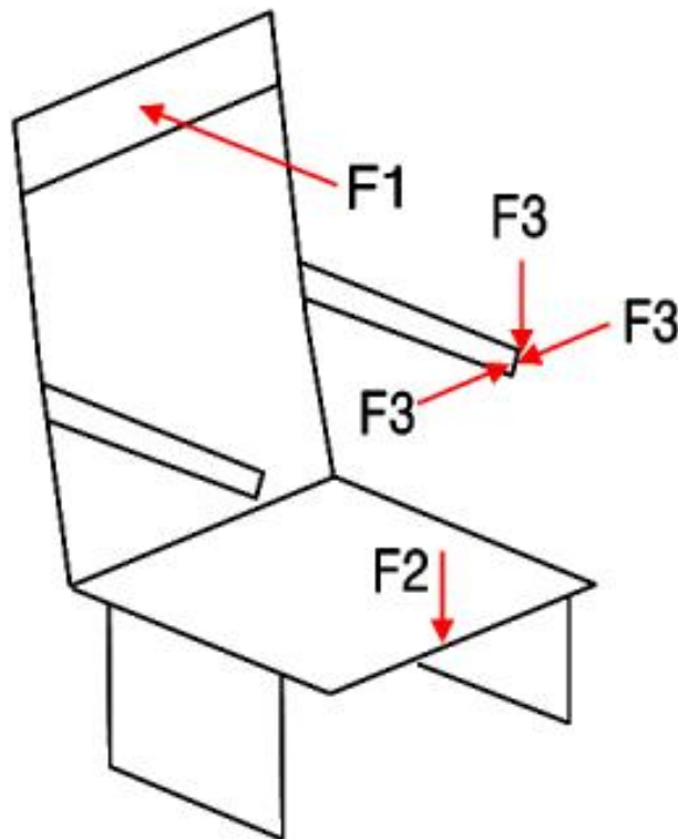
그림 1. 객실의자의 정하중 작용 기준
