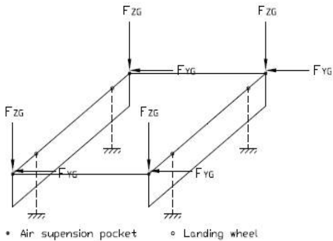
그림 4. 착지주행 좌우하중시험의 대차 고정 및 하중 부가
