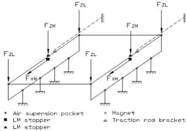
그림 9. 추진전동기 하중시험의 대차 고정 및 하중 부가
