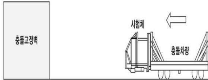
그림 1 고정벽 충돌시험 개략도
